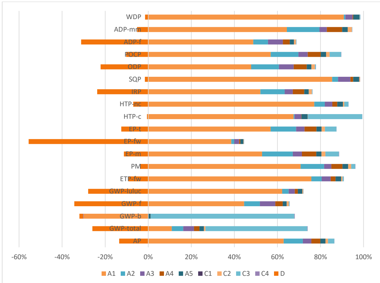
Figuur 2 Aandelen van de productlevensfasen in de milieueffecten voor Jumpax® HD
