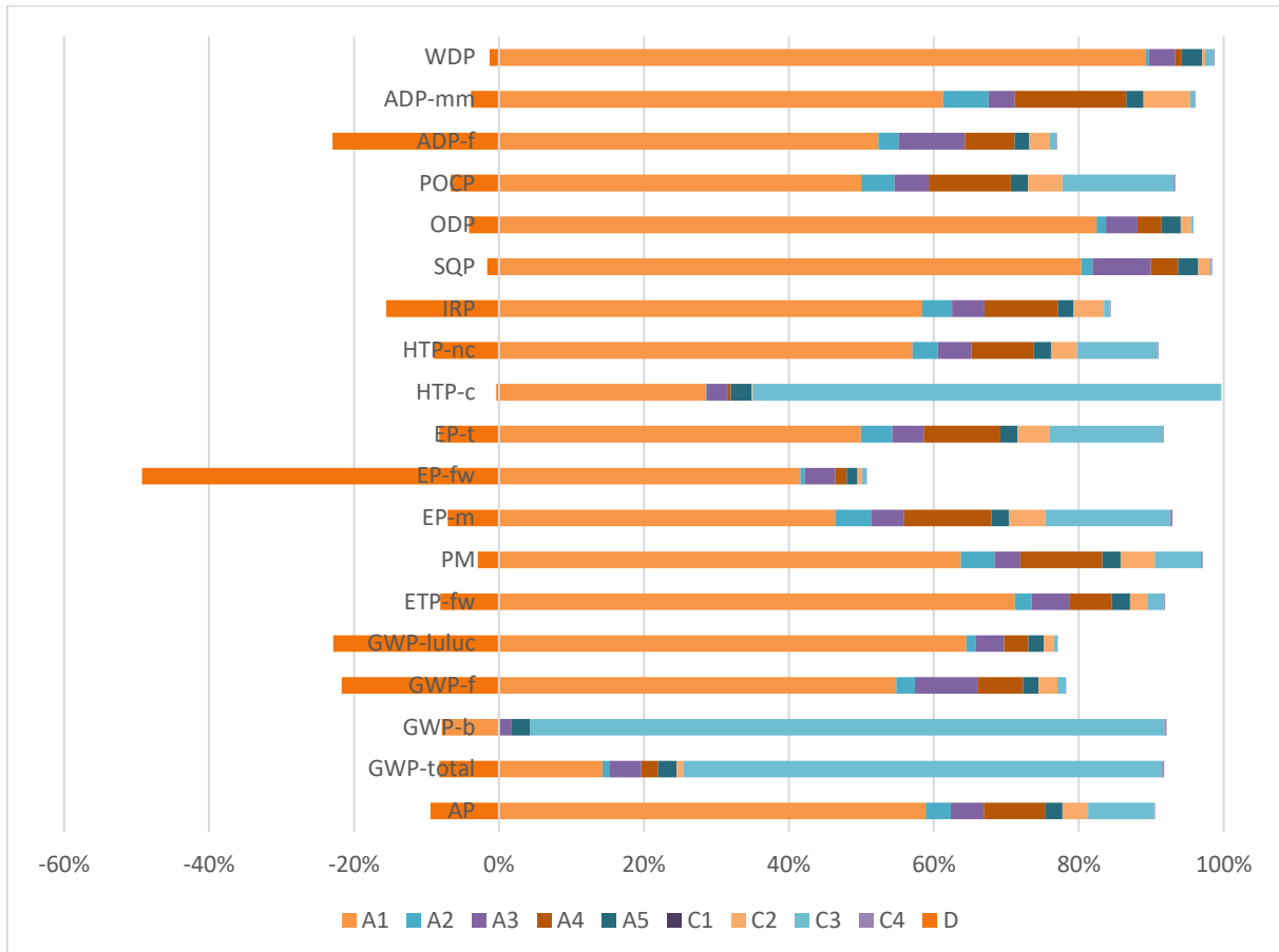
Figuur 2: Aandeel van de productlevensfasen in de milieueffecten voor Jumpax® Strong
